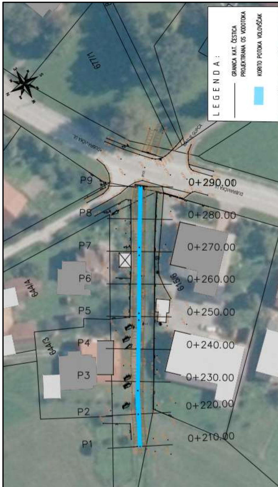
Slika 2.2-1. Situacijski prikaz zahvata na potoku Volovščak, stac. km 0+210 do stac. km 0+290 (izvor: Viacon, 2019.)
