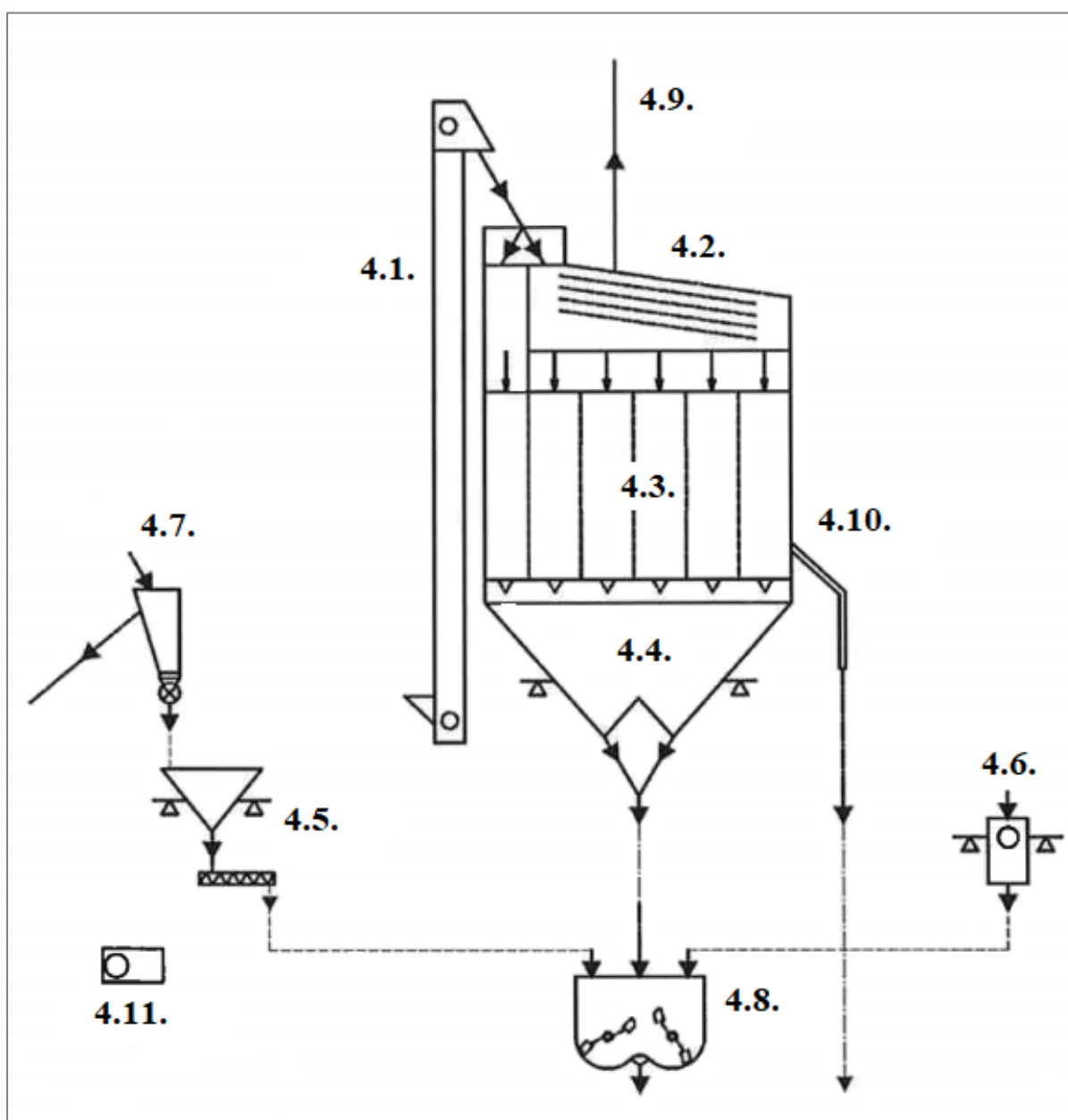
Slika 5. Shematski prikaz tijeka postupka miješanja
