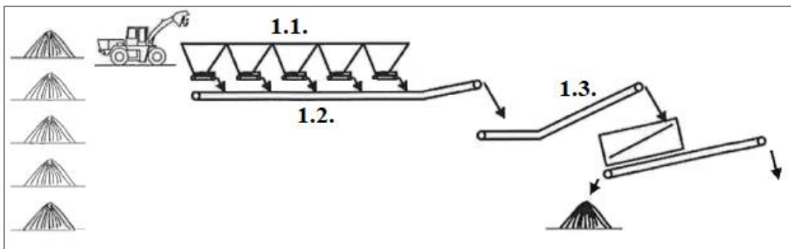
Slika 2. Shematski prikaz tijeka postupka predoziranja sa unosnom trakom
