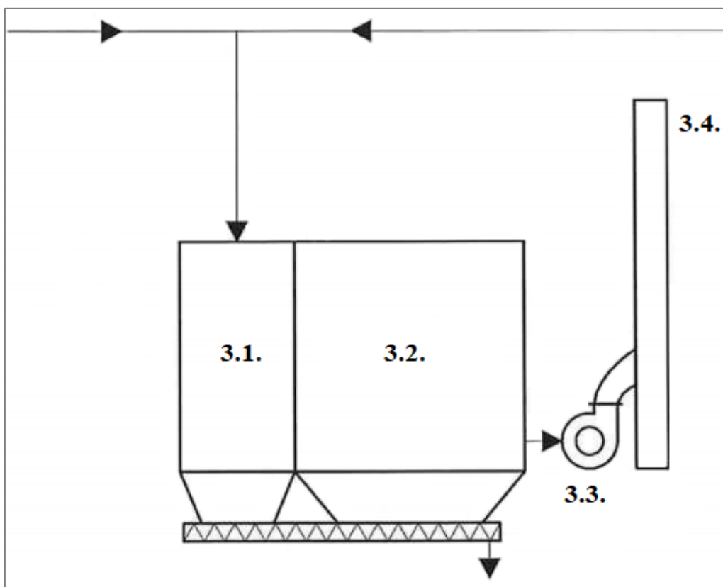
Slika 4. Shematski prikaz tijeka postupka otprašivanja
