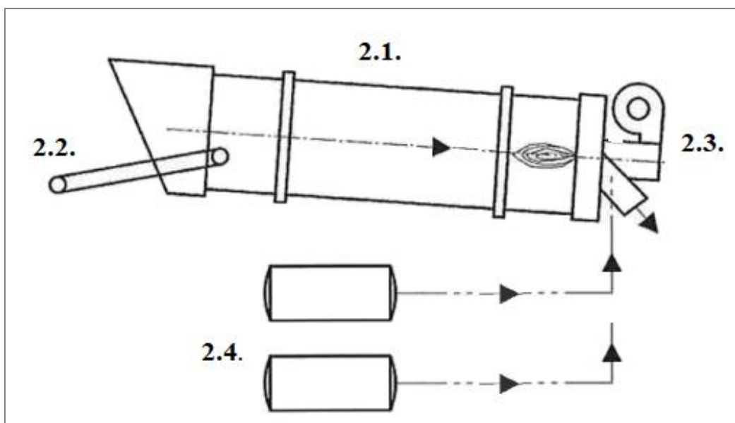
Slika 3. Shematski prikaz tijeka postupka s uređajem za sušenje te opskrbom istog lož uljem
